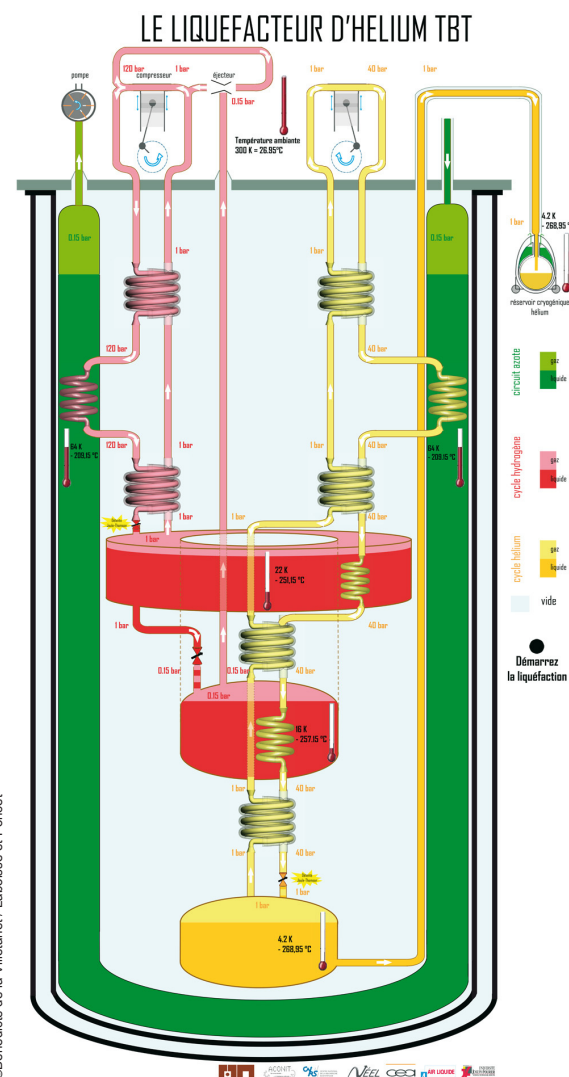
Panneau de démonstration permettant de simuler la liquéfaction.
